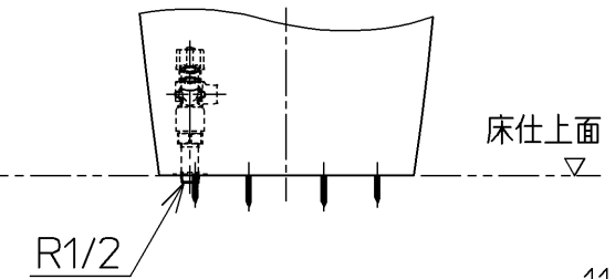
正面図
